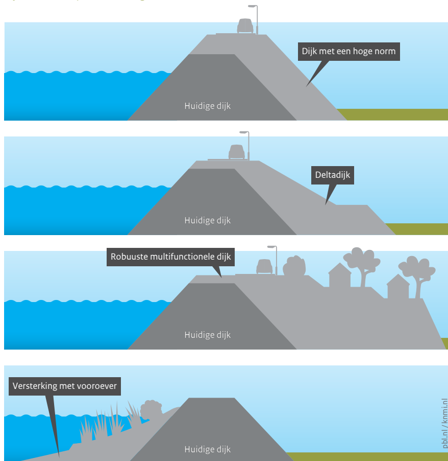
Figuur 2.10 Opties voor dijkversterking
