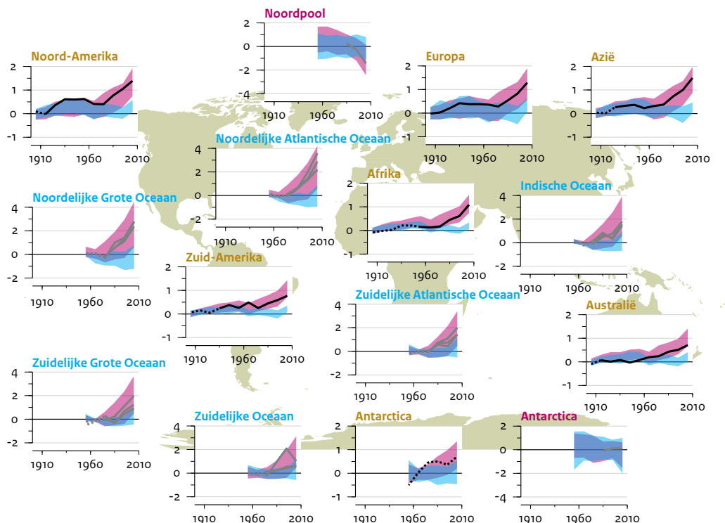
Figuur 1.5 Vergelijking van waargenomen en gemodelleerde klimaatverandering
