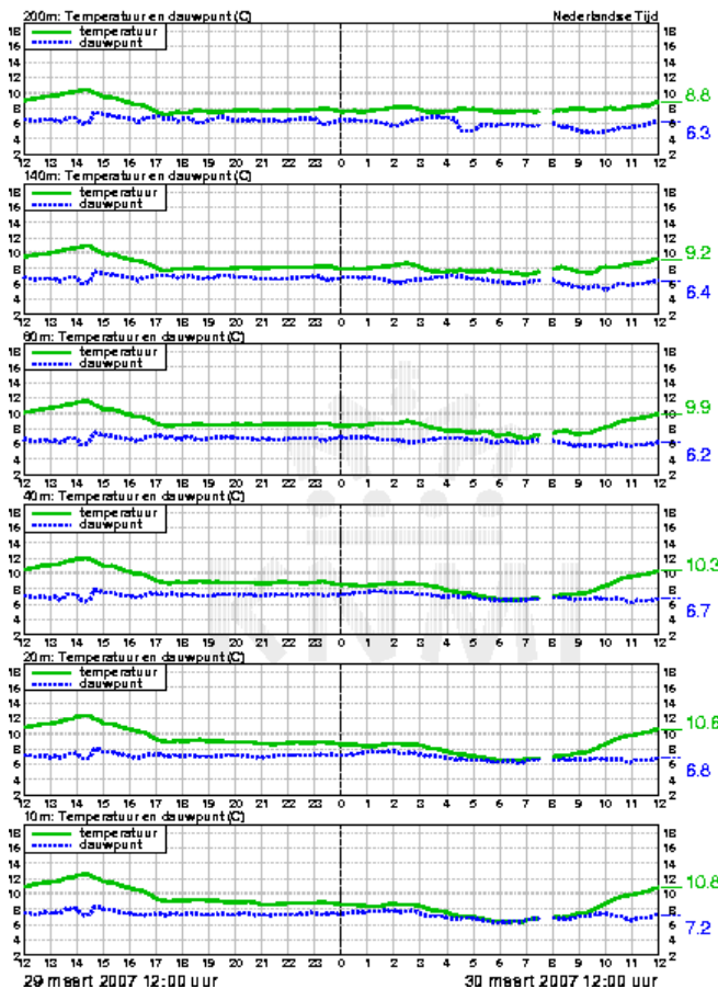
Figuur 11, lucht- en dauwpunttemperatuur, gemeten op de mast van Cabauw. Deze metingen geven tot 200 m hoogte informatie over het temperatuur en dauwpunt profiel.
