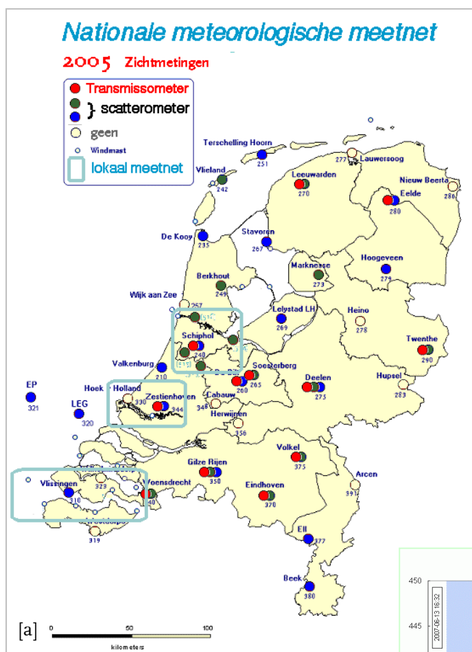
Figuur 2, overzicht van de posities van zichtmeters op land ([a]; situatie 2005) en op zee ([b]; gepland en gerealiseerd); voorzien is de plaatsing van zichtmeters op de stations Westdorpe, Wilhelmina- dorp en Herwijnen. Aangeduid zijn de lokale meetnetten "Mist- posten Schiphol, Mistmeetnet van het GhR en het "Mistmeet Zeeland", zie [c], BTP, [d] RNW en [e] ZLD.
