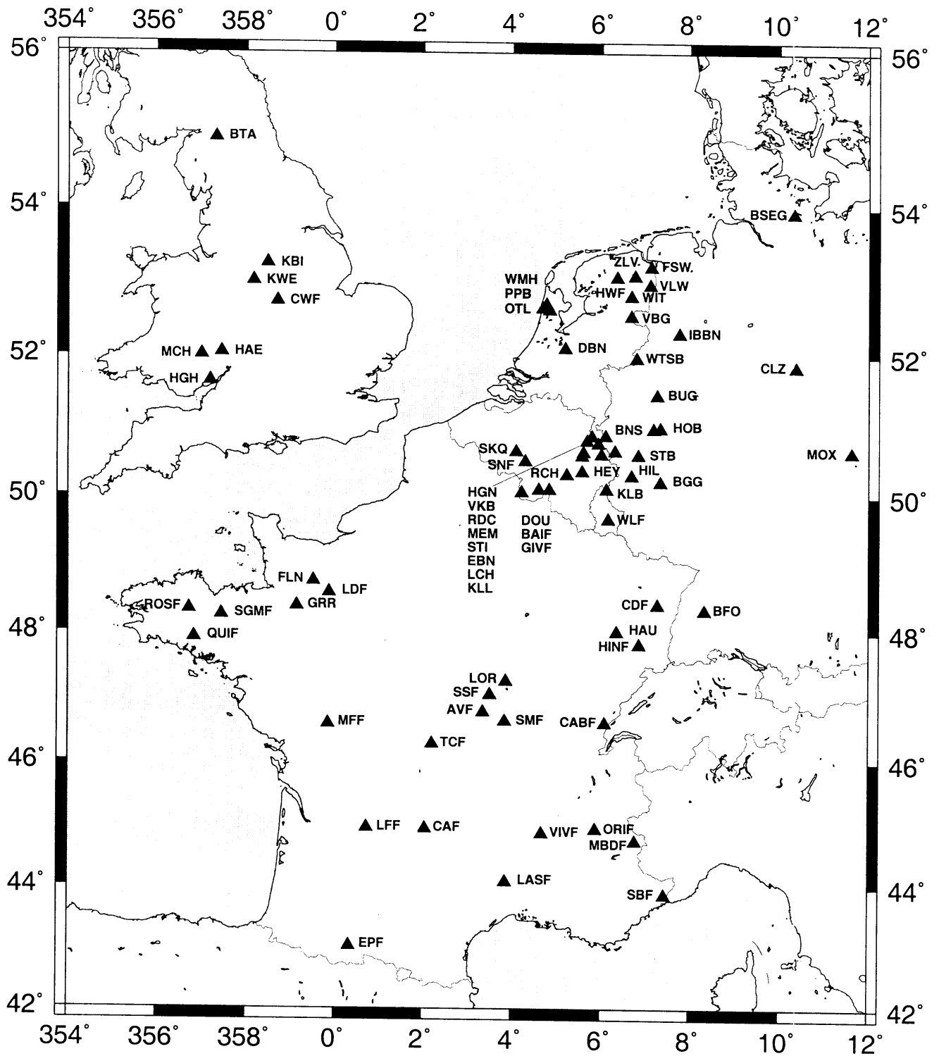
Figuur 1. Overzicht van de seismische stations die de aardbeving bij Alkmaar van 9 september 2001 geregistreerd hebben.
