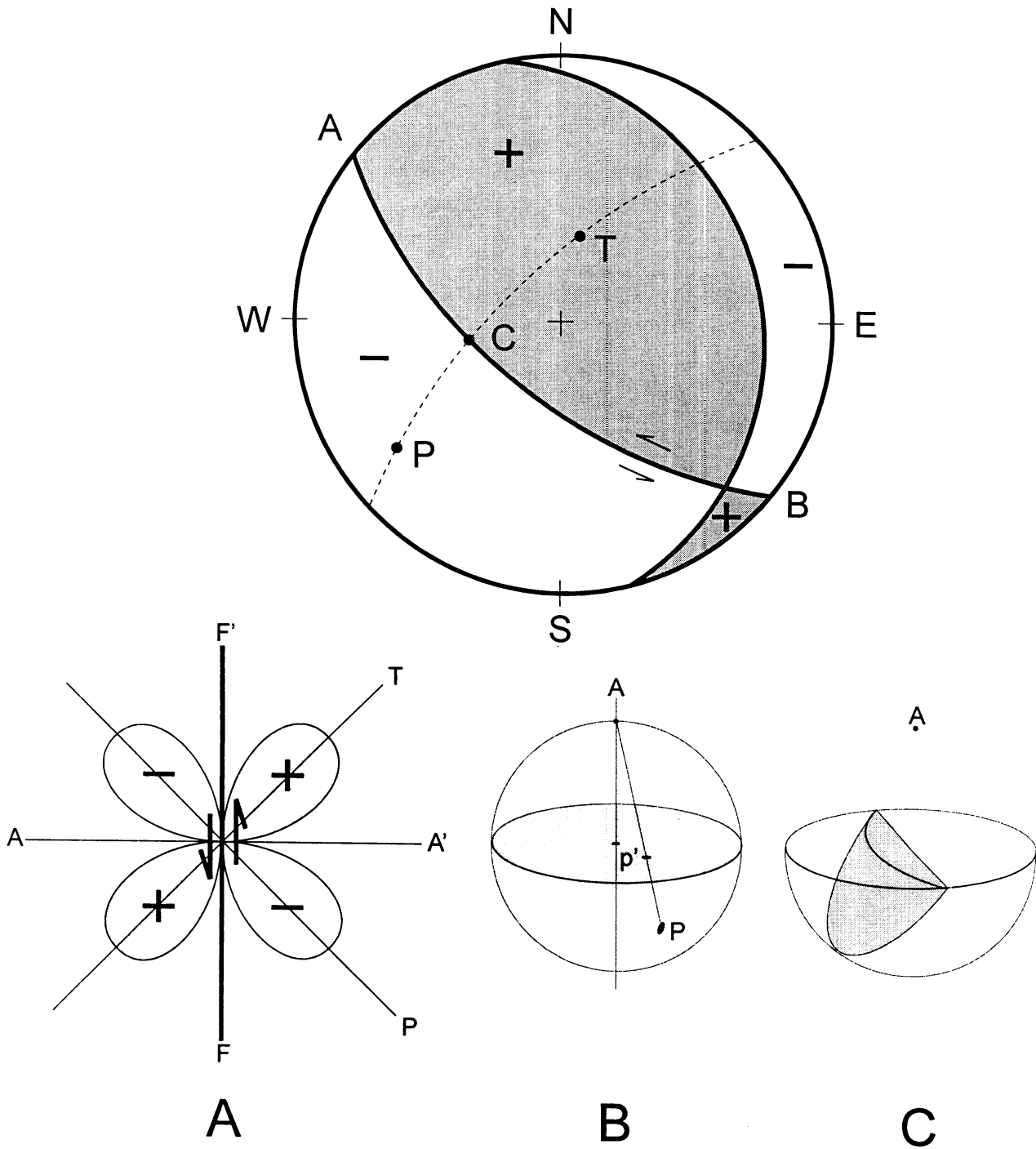
Figuur 5. Haardoplossing van de twee bevingen bij Alkmaar op 9 en 10 september. De representatie is een stereografische projectie van het breukvlak (zie figuur B). Een vlak wordt in deze representatie als een cirkelboog weergegeven (zie figuur C). Het stralingspatroon van de P-golven heeft in verschillende richtingen een verschillend teken (zie figuur A). In de bovenste figuur is de lijn ACB de projectie van het breukvlak op de onderbol. C is de projectie van de slipvector in het breukvlak. P en T zijn de projecties van respectievelijk de druk- en de rek-as. Het + teken geeft compressie weer in het stralingspatroon van de P-golven, het - teken de dilatatie. Het mechanisme komt overeen met een overschuivende breuk met een hellingshoek van 66^\circ en een strekking van 130^\circ . Er is een kleine linkslaterale component zichtbaar.
