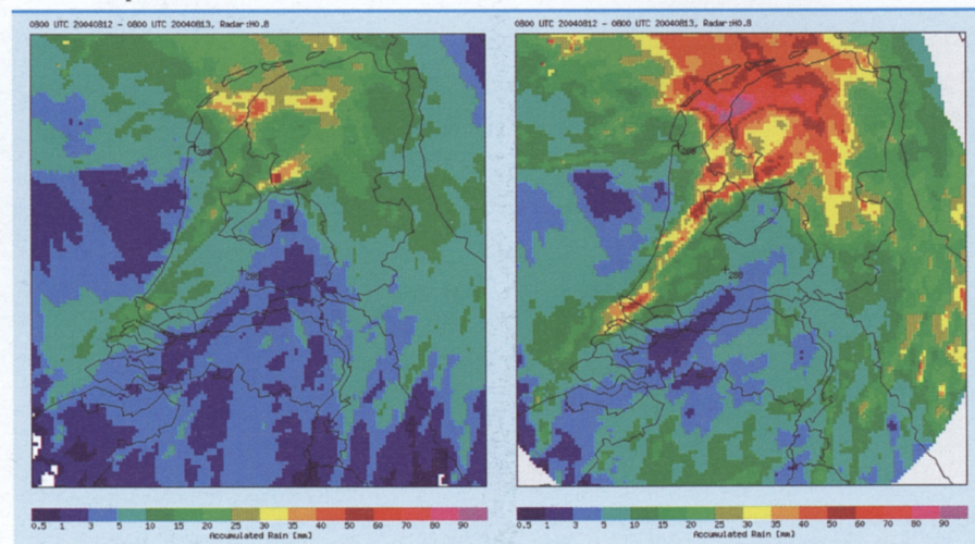
Afb. 1: De ruwe (links) en gecorrigeerde (rechts) radaraccumulaties voor de periode van 08.00 uur op 12 augustus tot 08.00 uur op 13 augustus 2004. De correctie is uitgevoerd met de neerslaganalyse van Holleman 3) en gebaseerd op Michelson 6) .
