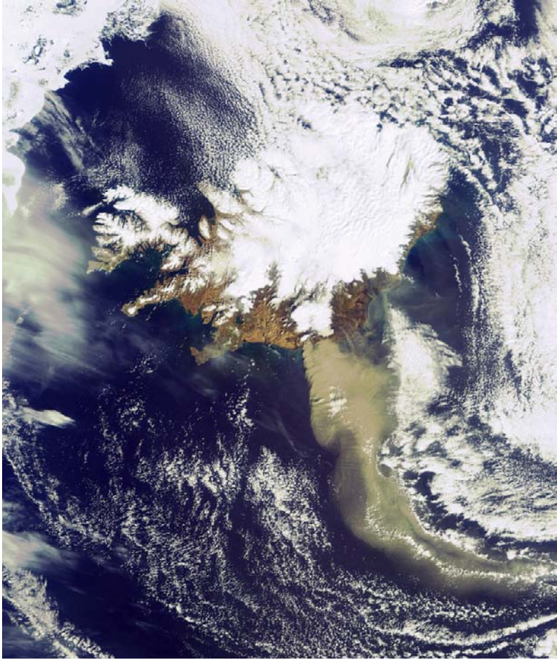
Figuur 1.4: Satellietfoto van IJsland en omgeving op 19 april 2010. De contouren van IJsland en de bruine pluim van vulkanisch materiaal, afkomstig van de Eyjafjallajökull, zijn duidelijk zichtbaar (Bron: ESA, MERIS instrument aan boord van ENVISAT).
