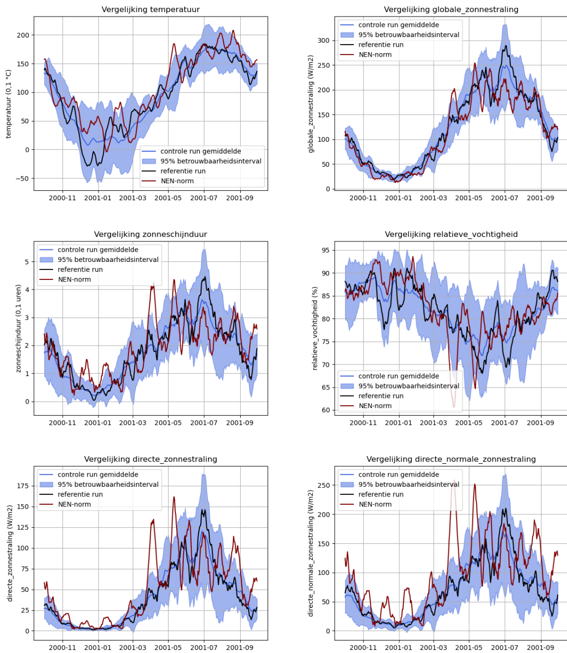
Figuur 10: Klimaatjaar voor de warmtevraag voor temperatuur, globale straling, zonneschijnduur, relatieve vochtigheid, directe straling en directe normale straling volgens de NEN5060 norm (paars) en het gemiddelde van alle 15 controle RACMO klimaten (bruine lijn). De groene lijn geeft het gekozen klimaatjaar aan voor de referentie periode. De shading geeft de 95% onzekerheidsband aan die volgt uit de 15 controle klimaten.
